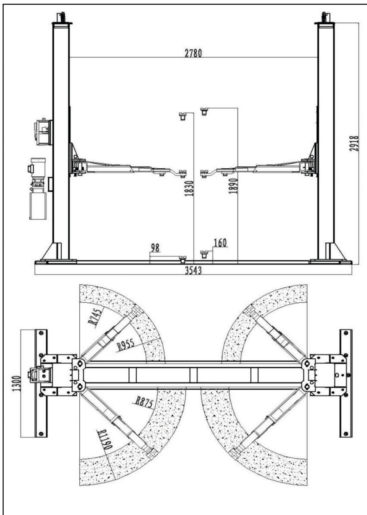
Figure 1 (Dimensions de le pont élévateur)
